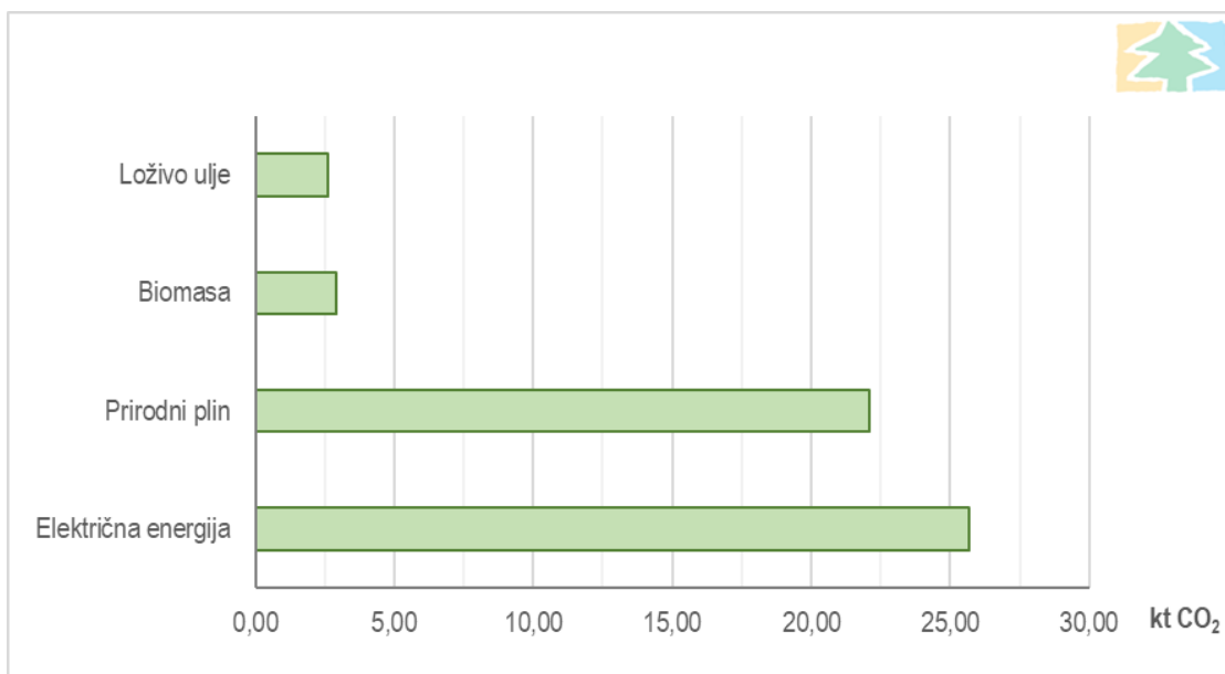
Slika Pogreška! U dokumentu nema teksta navedenog stila..10 Procijenjene količine emisija CO 2 iz sektora kućanstva u Požeško-slavonskoj županiji u 2020. godini (Izrađivač: IRES EKOLOGIJA d.o.o.)
